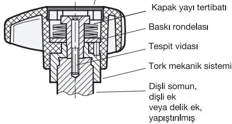
Plastik kapak
